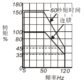
基本频率50Hz(V/F:50Hz用) (电压: 220V)
