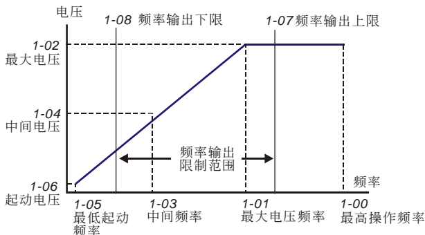
V/F曲线
