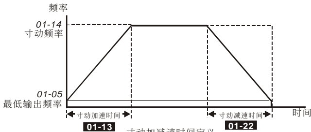
寸动加减速时间定义
