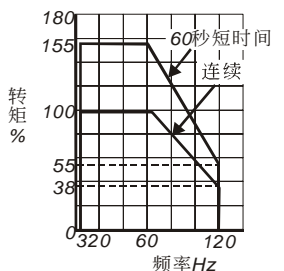
基本频率60Hz(V/F:60Hz用) (电压: 220V)
